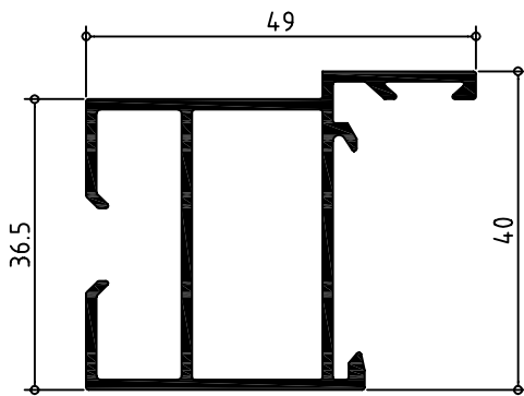
082620 HOJA SIN JUNQUILLO
