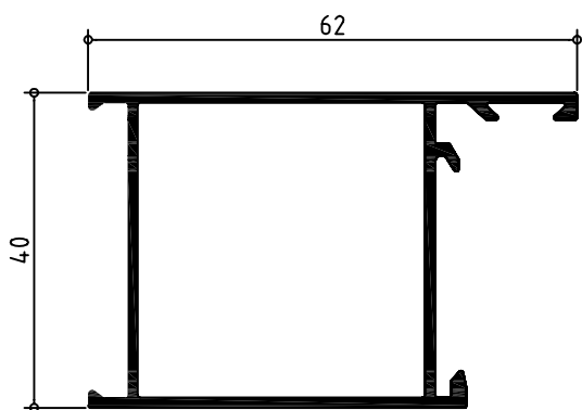
440140 CERCO 40 X 40
