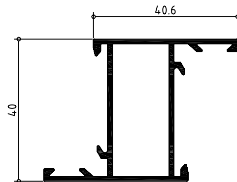
420340 HOJA 40 X 20
