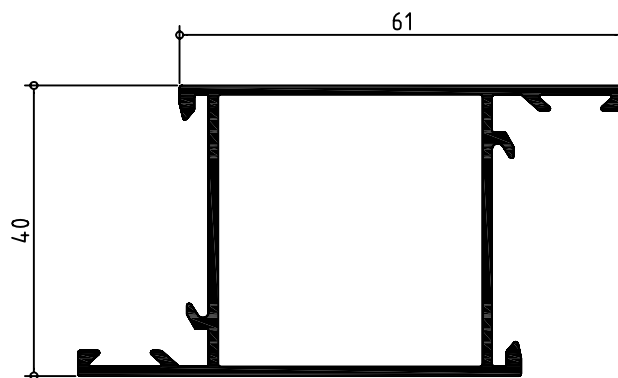
440340 HOJA 40 X 40
