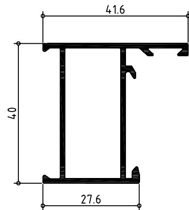
420140 CERCOS 40 X 20
