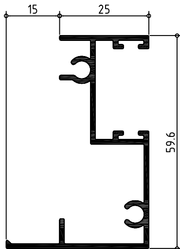
072573 MARCO LATERAL SOLAPE IZQDO
