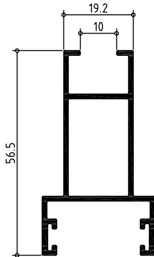
072285 HOJA CENTRO TOPE
