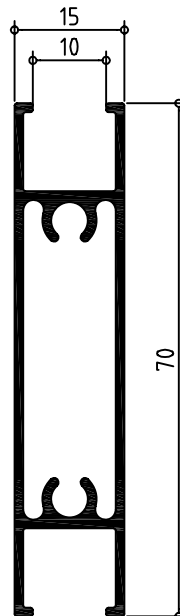
072910 ZOCALO CENTRO H.10
