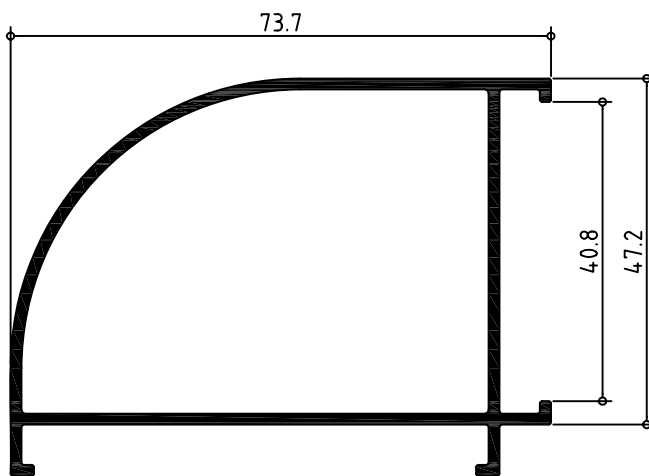
600172 ESQUINERO MIXTO ABATIBLE CORREDERA
