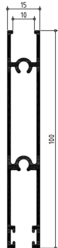
072900 ZOCALO BAJO H.10
