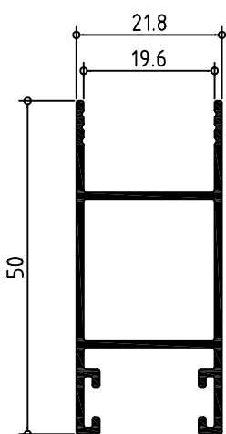
121325 HOJA LATERAL CLIMALIT 50
