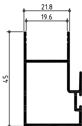
121261 HOJA CENTRO CLIMALIT 45
