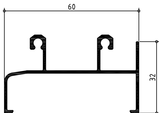
121185 GUIA INFERIOR ABIERTA
