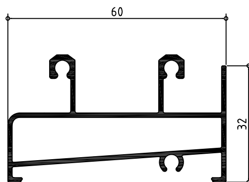
121186 GUIA INFERIOR TUBULAR
