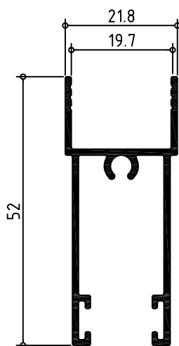
121360 HOJA RUEDAS CLIMALIT
