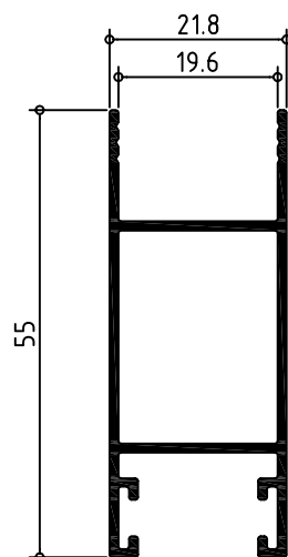
121320 HOJA LATERAL CLIMALIT 55
