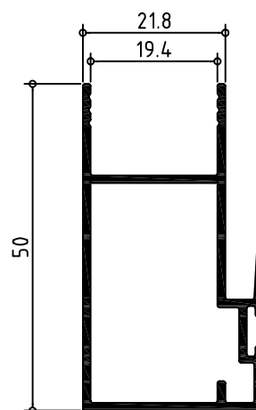
121262 HOJA CENTRO CLIMALIT 50
