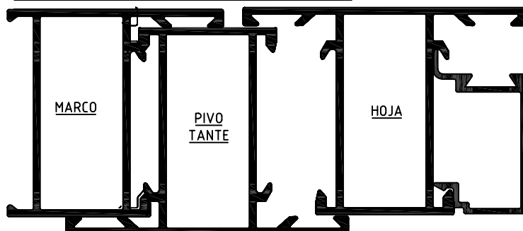
CORTE SECCION ANCHO LATERAL DCHO. INFERIOR EL PERFIL PIVOTANTE VA COGIDO AL MARCO
