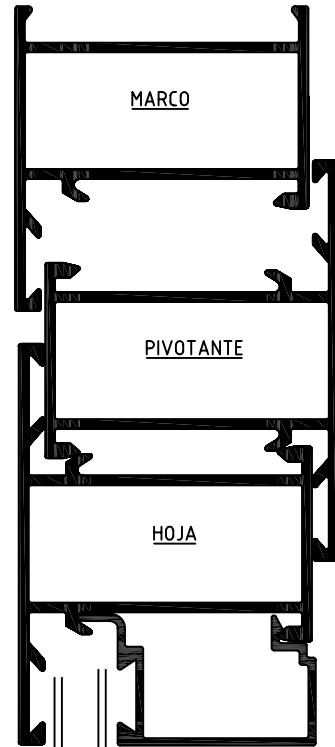
CORTE SECCION ALTURA TOTAL
