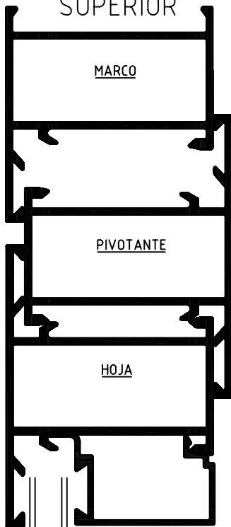
CORTE SECCION ANCHO SUPERIOR
