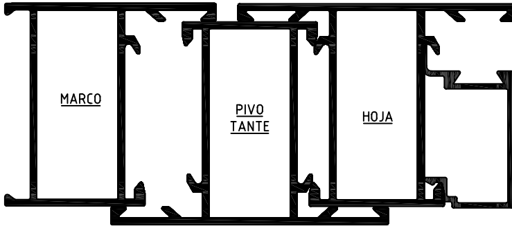
CORTE SECCION ANCHO LATERAL IZDO. SUPERIOR EL PERFIL PIVOTANTE VA COGIDO A LA HOJA
