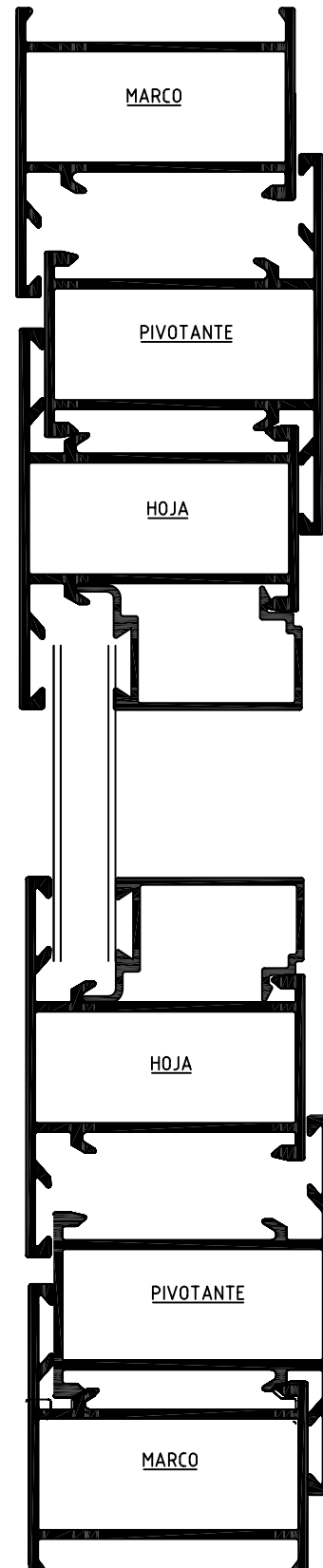
CORTE SECCION ALTURA TOTAL
