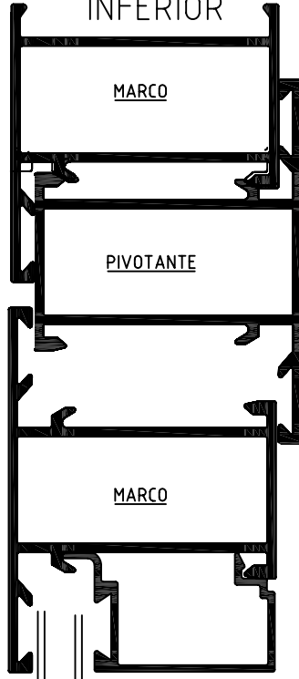
CORTE SECCION ANCHO INFERIOR
