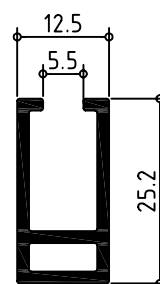
073997 PERFIL TAPALUZ
