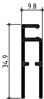
073995 PERFIL MOSQUITERO
