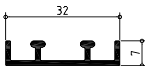
065165 GUIA INFERIOR
